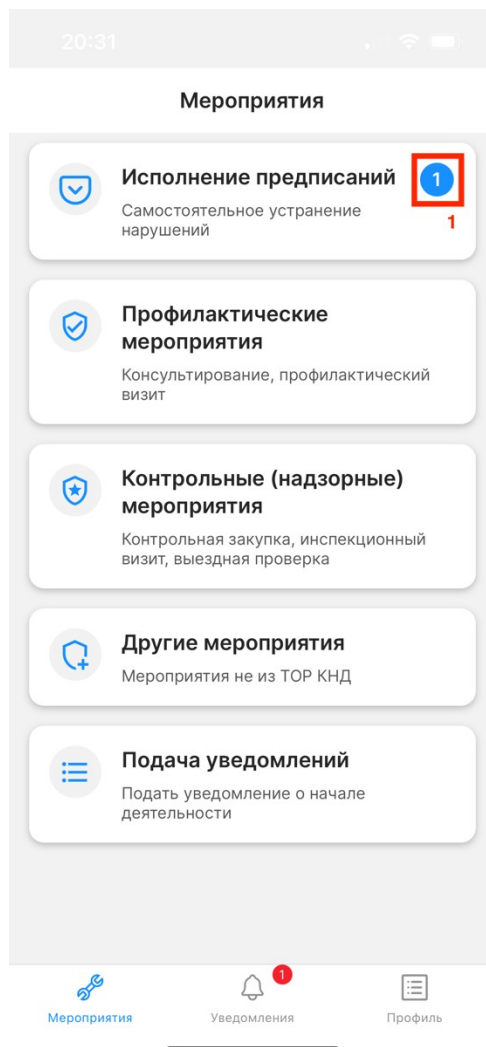
Рисунок 45. Исполнение предписаний
